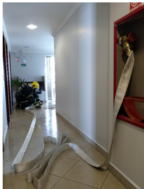
Adutora conectada do hidrante ao divisor
